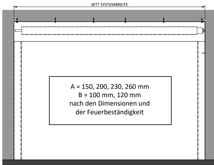
GEBÄUDEPLAN - MONTAGE IN DER ÖFFNUNG
