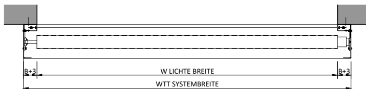
GEBÄUDEPLAN - MONTAGE AN DIE WAND
