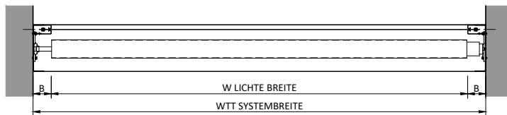
GEBÄUDEPLAN - MONTAGE AN DIE WAND
