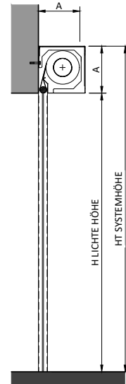
SCHNITT WANDMONTAGE
