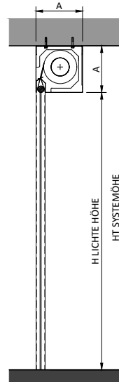
SCHNITT ÖFFNUNGSMONTAGE
